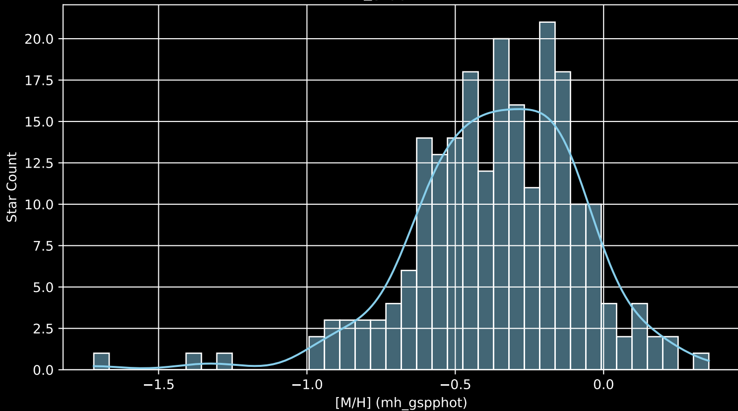
GALAH DR4 Field: [8488] [M/H] (mh_gspphot) (n= 219)
