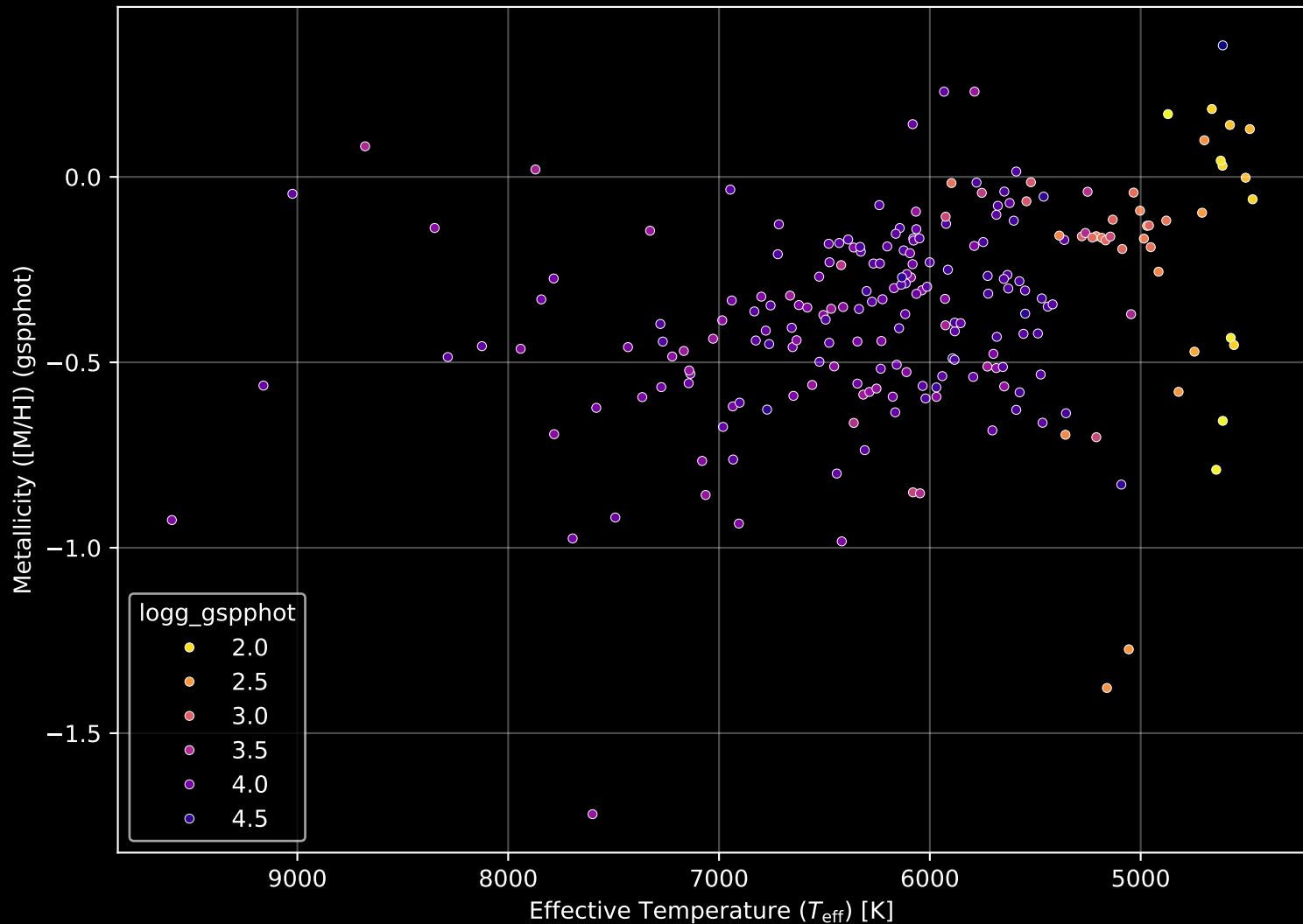
GALAH DR4 Field: [8488] Stellar Population Parameters (n= 219)
