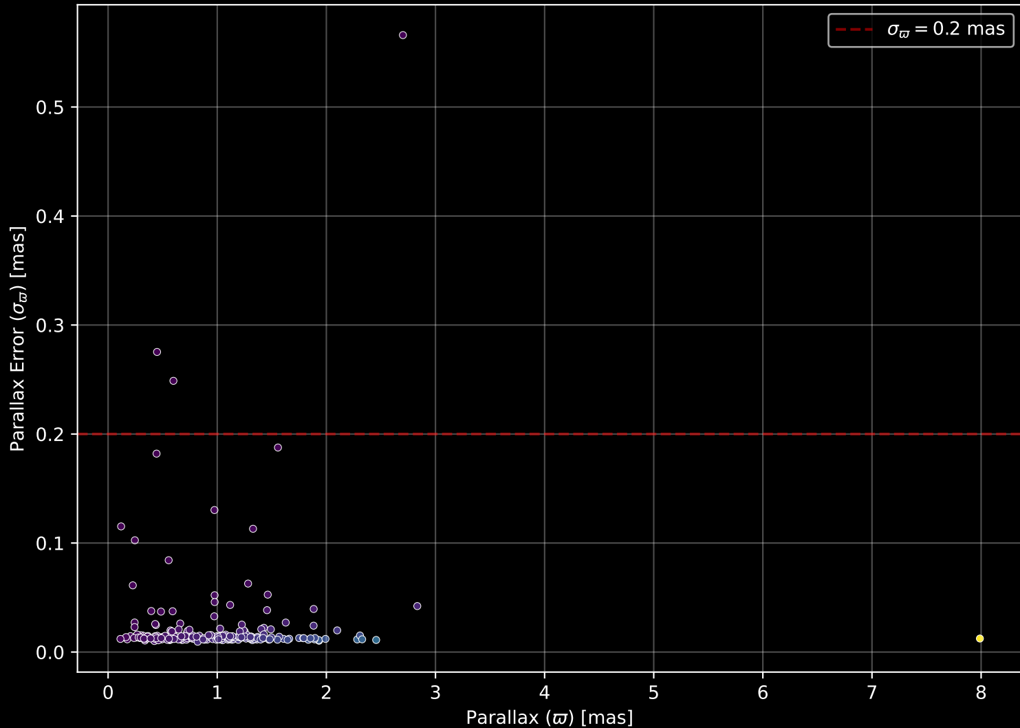
GALAH DR4 Field: [8488] Parallax Quality (n= 219)
