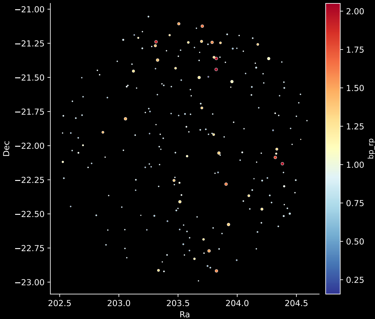
GALAH DR4 Field: [8488] Stars: 219
